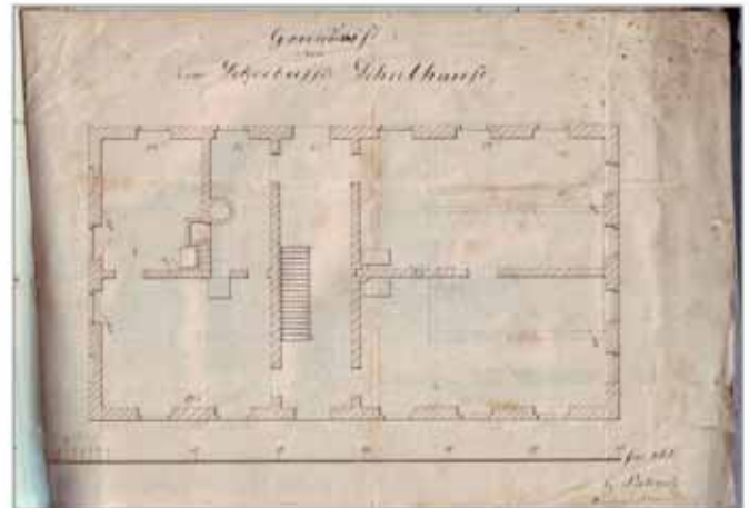
Grundriss des Schulneubaus von 1854, gezeichnet vom Drebkauer Maurermeister G. Pahms; links die Lehrerwohnung, rechts die Klassenzimmer.
